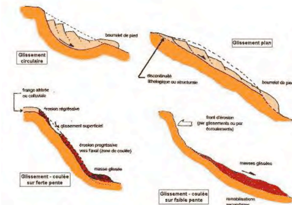
Différents glissements de terrain (Géorisques)
