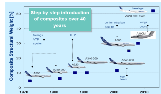
Structures Avions, les Tendances d'Evolution Compétition : Métal / Composite
